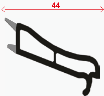
70 mm Tek Cam Çıtası
