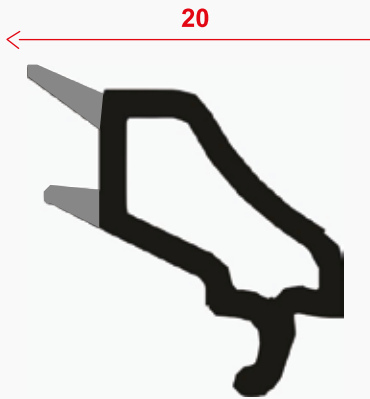
60 mm Çift Cam Çıtası
