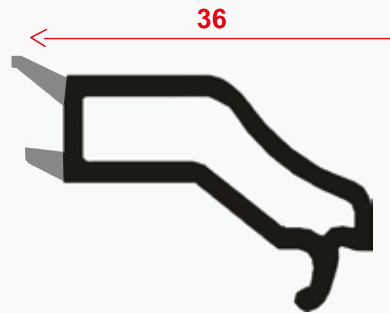
60 mm Tek Cam Çıtası
